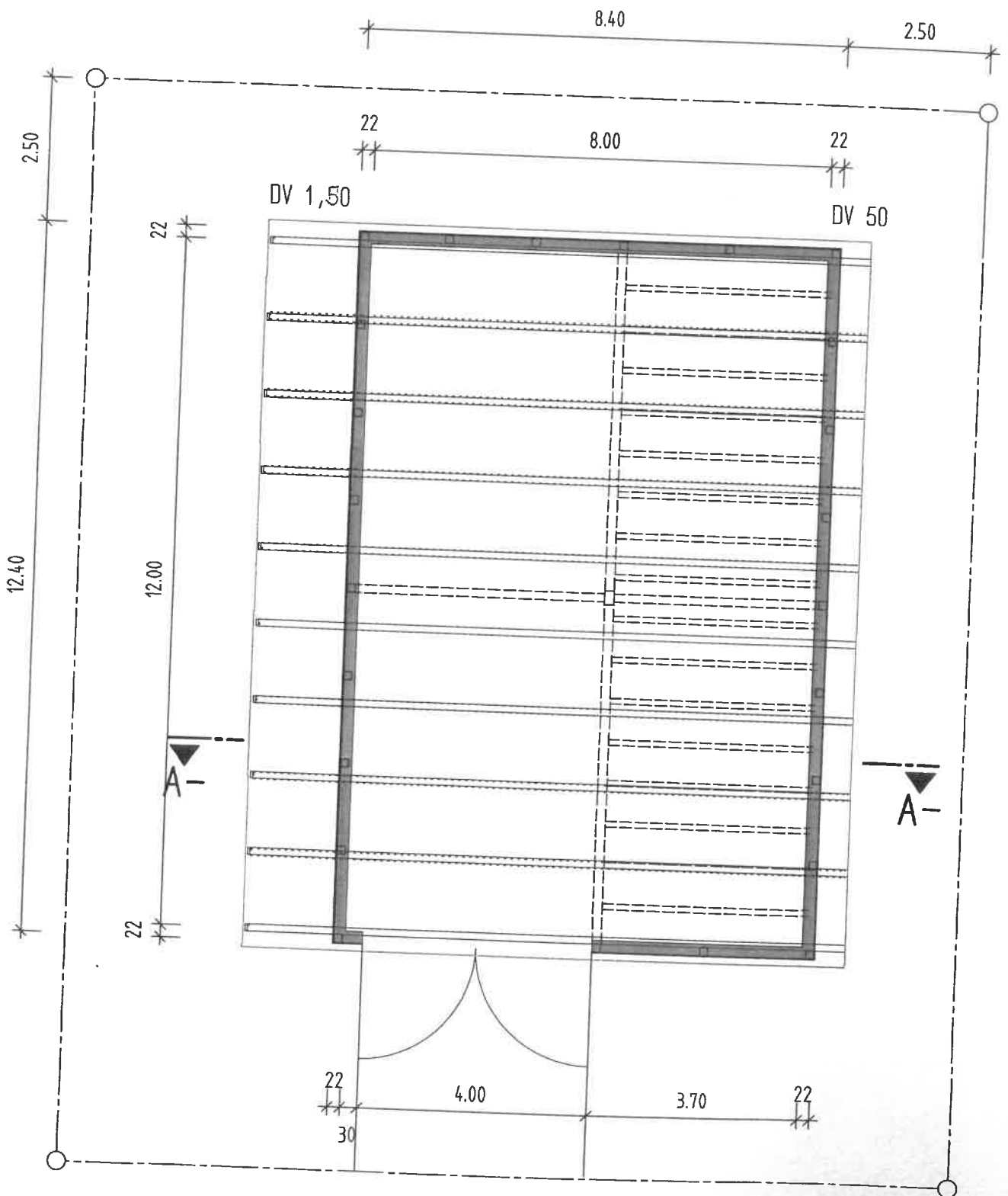
GRUNDRISS
